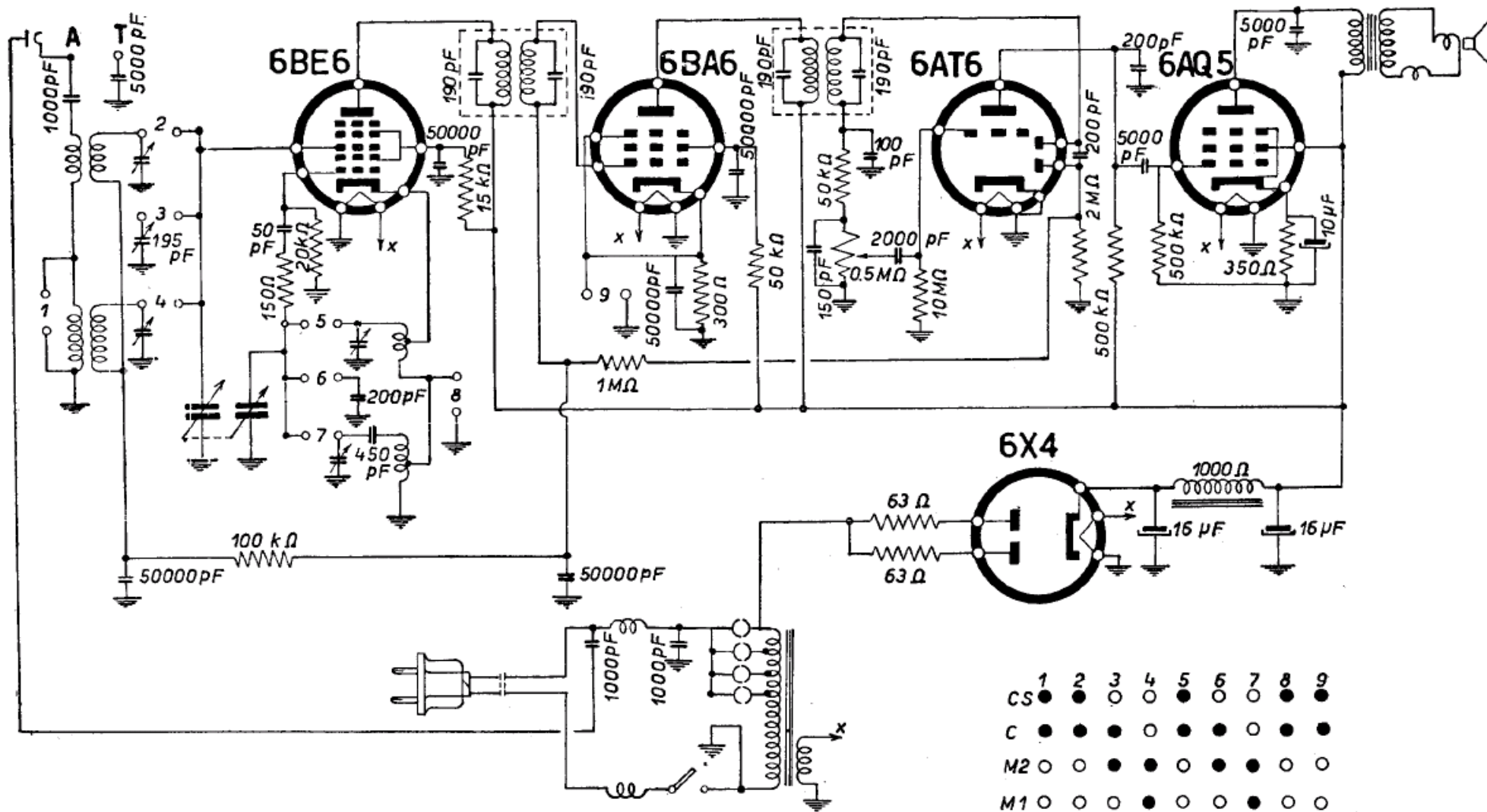
PHONOLA RADIO - Mod. 577 D - Con valvole miniatura. Gamma onde medie e gamma onde corte ciascuna con semigamma spostata. Media frequenza 470 kc. Potenza d'uscita 1,5 W.
